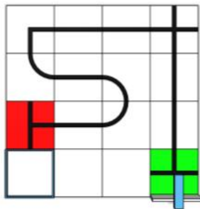
Рис. 3. Возможный вариант расположения ячеек поля: зелёная ячейка – ячейка получения шариков с устройством выдачи шариков, красная ячейка – ячейка выгрузки шариков, в нижнем левом углу – место складирования шариков.
